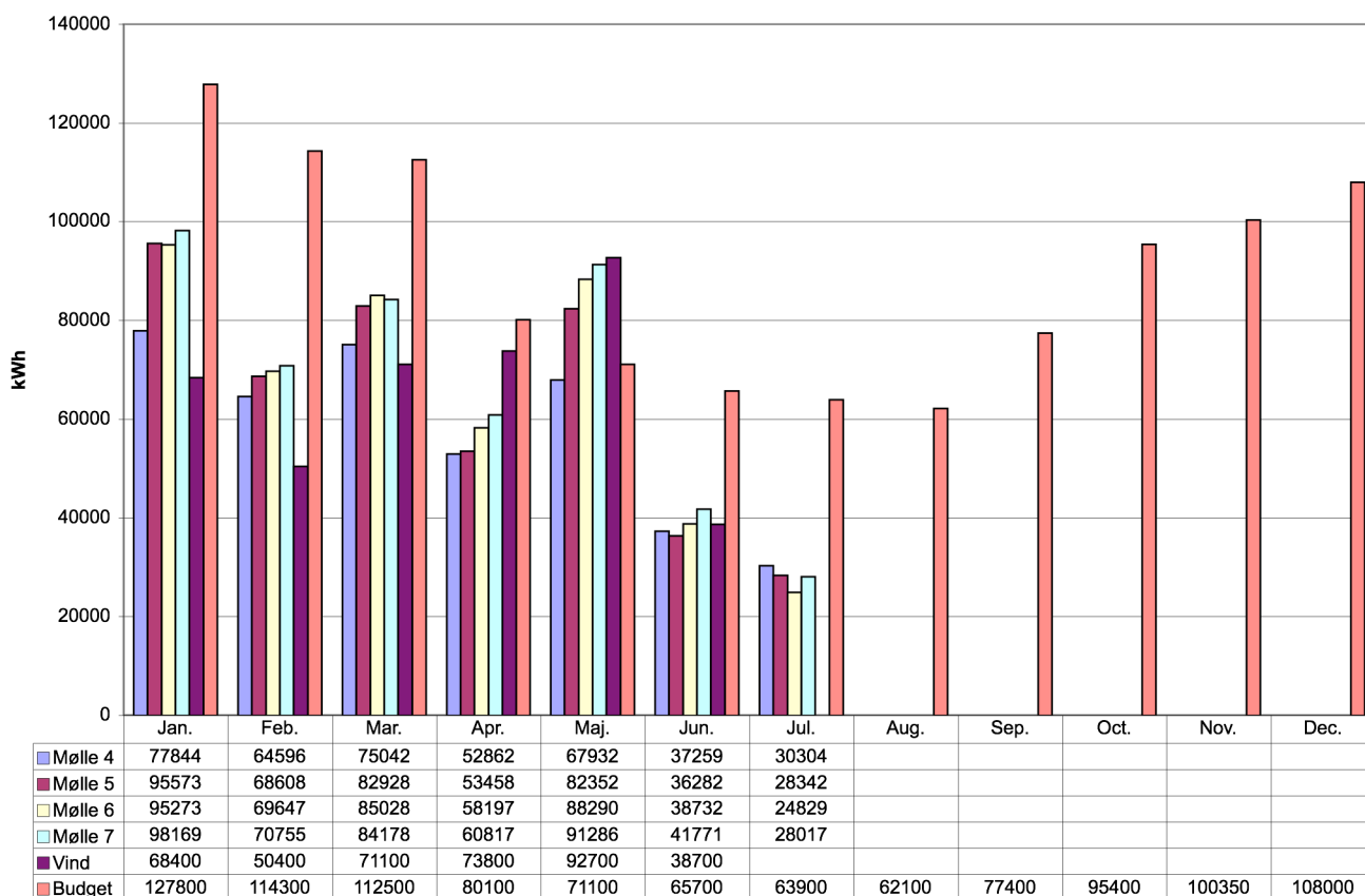
Lynetten Vindkraft Produktion 2006
